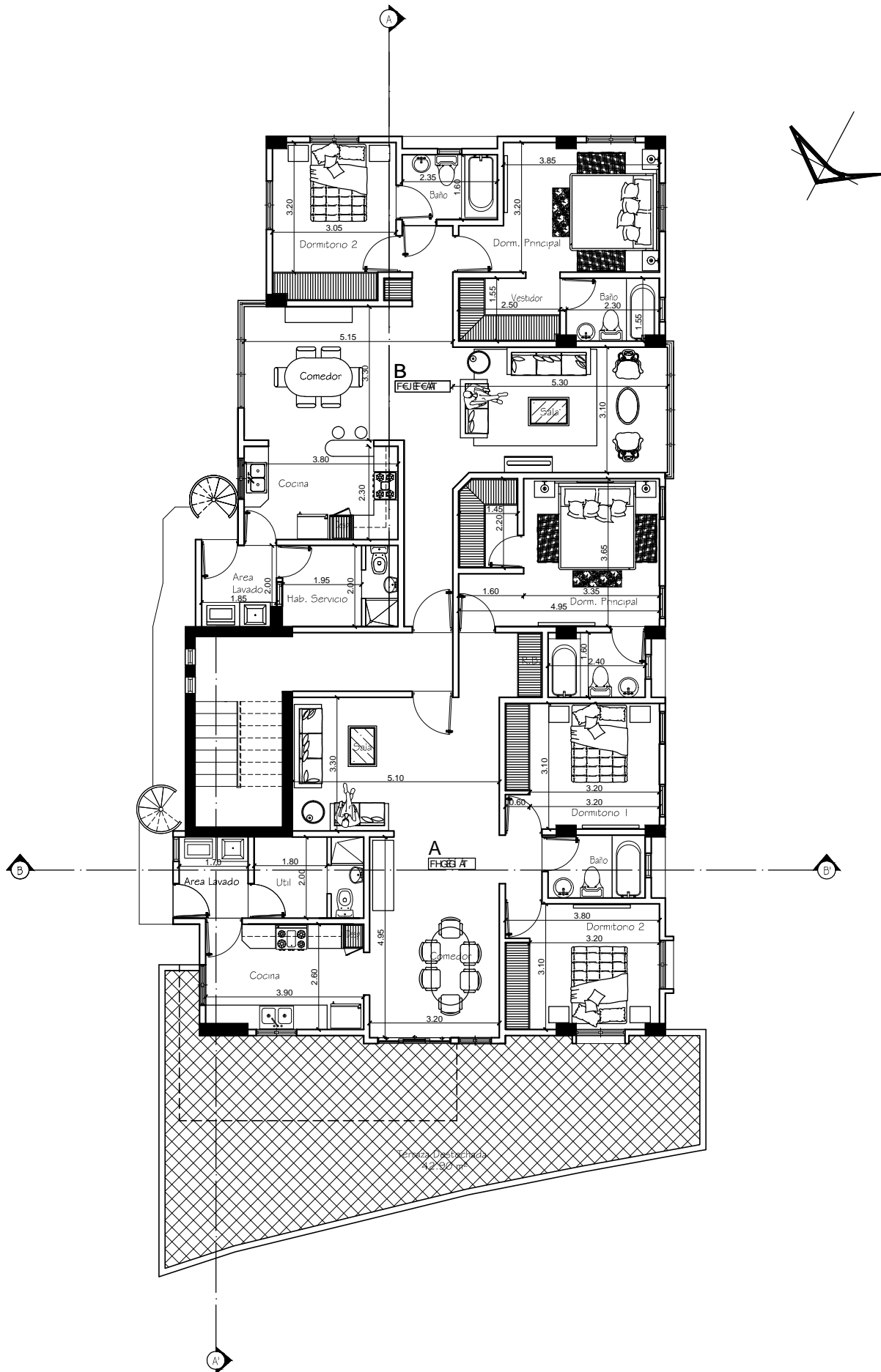
PLANTA ARQUITECTONICA AMUEBLADA 2DO. NIVEL APARTAMENTOS
