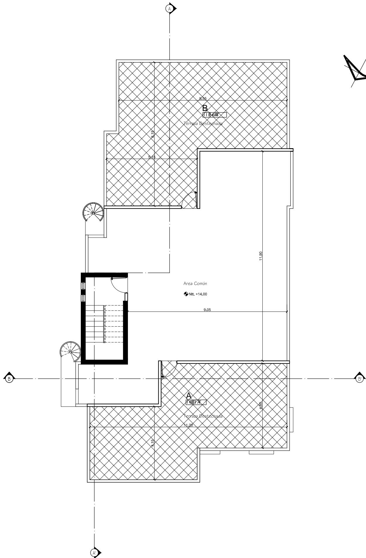
PLANTA ARQUITECTONICA AMUEBLADA 6TO. NIVEL (TERRAZA)
