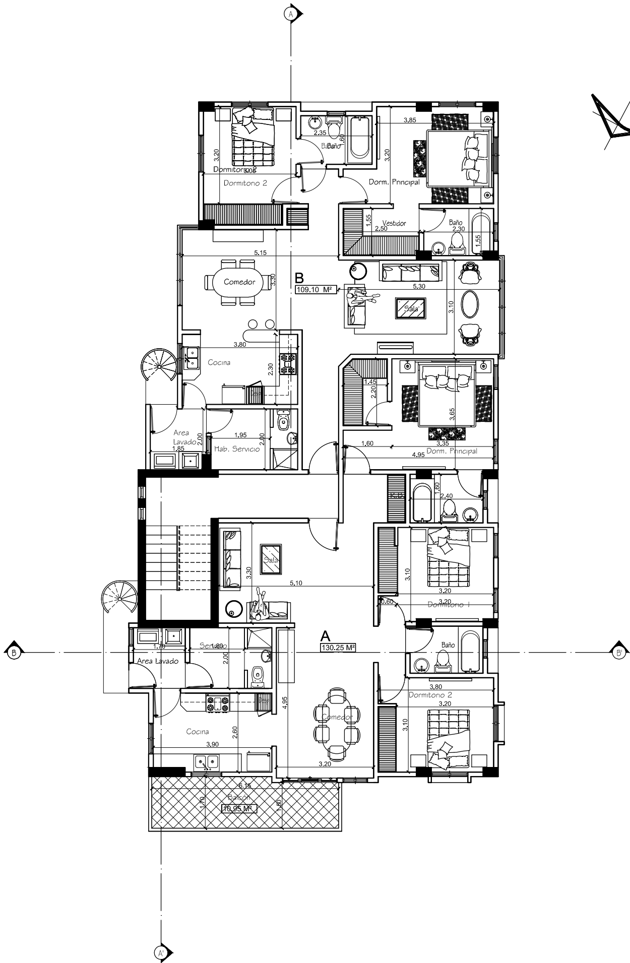
PLANTA ARQUITECTONICA AMUEBLADA 4TO. Y 5TO. NIVEL APTOS.
